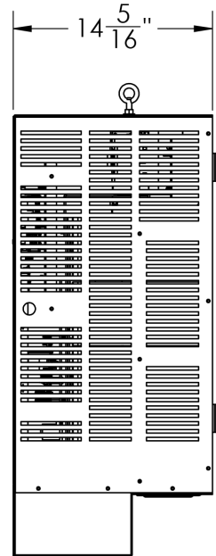
SIDE NEMA 1
