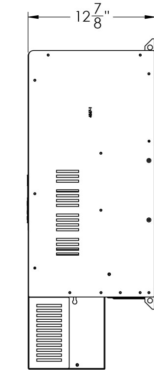
SIDE NEMA 1
